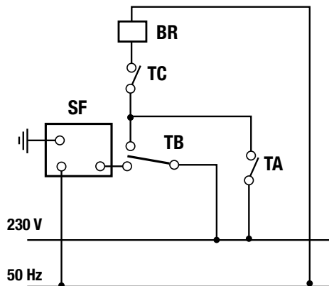
Schema di collegamento elettrico Electrical wiring diagram
