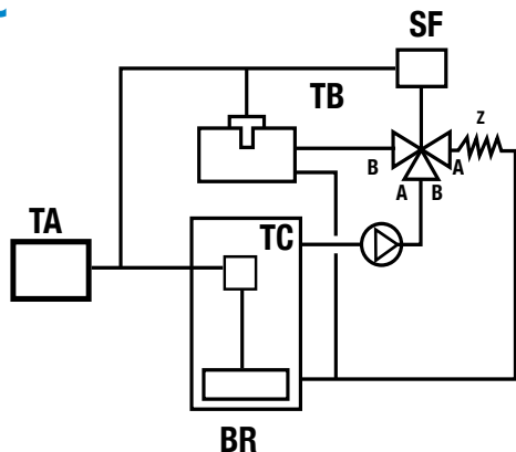
Esempio di applicazione precedenza bollitore Application example giving priority to the hot water heater
